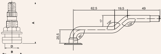
5. Metalen tubeless ventiel 6. Drievoudig gebogen universeel ventiel
